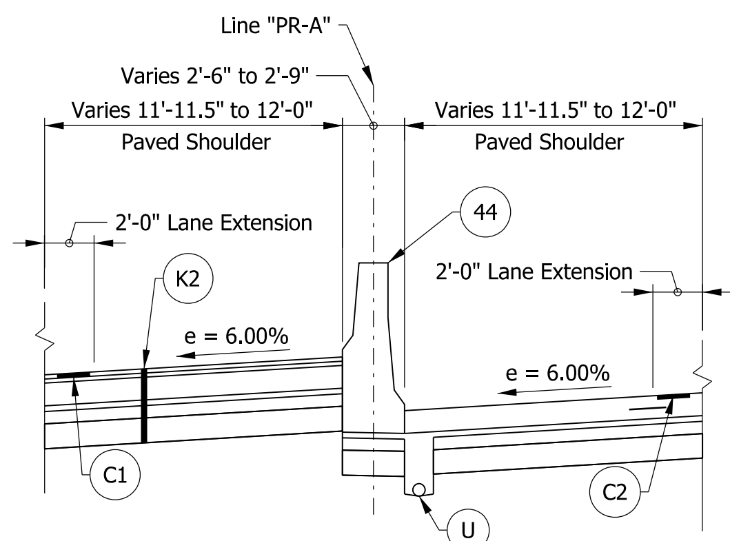
MODIFIED MEDIAN BARRIER DETAIL STA. 872+72.00 "PR-A" to STA. 873+02.00 "PR-A" STA. 878+98.00 "PR-A" to STA. 879+18.00 "PR-A" STA. 892+21.00 "PR-A" to STA. 892+41.00 "PR-A" STA. 894+57.00 "PR-A" to STA. 894+77.00 "PR-A"
